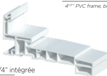
#9600MD Cadre 4 1/2" avec moulure à brique intégrée 4 1/2" PVC frame, built-in brick moulding
