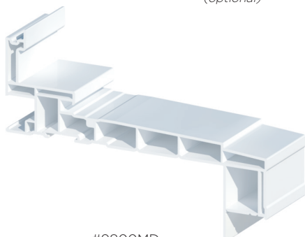
#9800MD Cadre en PVC avec moulure à brique intégrée 5 5/8" (structurale seulement) 5 5/8" PVC frame, built-in brick moulding (Structural only)
