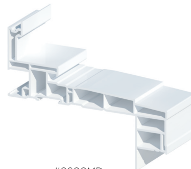
#9600MD Cadre 4 1/2" avec moulure à brique intégrée 4 1/2" PVC frame, built-in brick moulding
